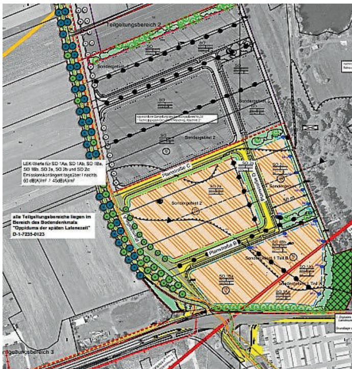
Lageplan zum Satzungsbeschluss zum Bebauungsplan Nr. 20 „Technologiepark Ost“
